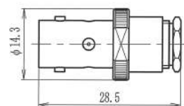
BNC-J-58U
