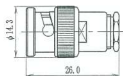
UG-88/U
