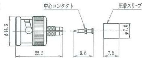
BNC-GP3-55U
