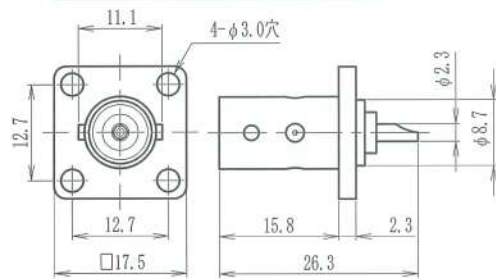
BNC-R
