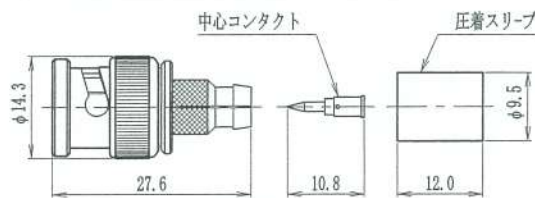
BNC-GP-5C
