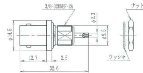
UG-657/U
