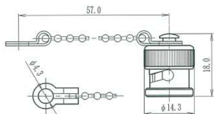
BNC-JC
