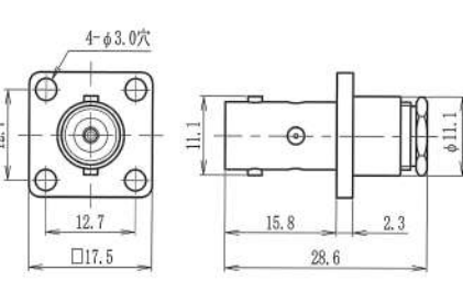
BNC-PJ-58U
