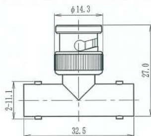
UG-274/U
