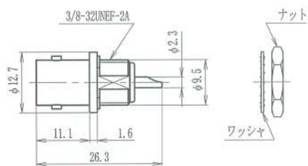
UG-625/U
